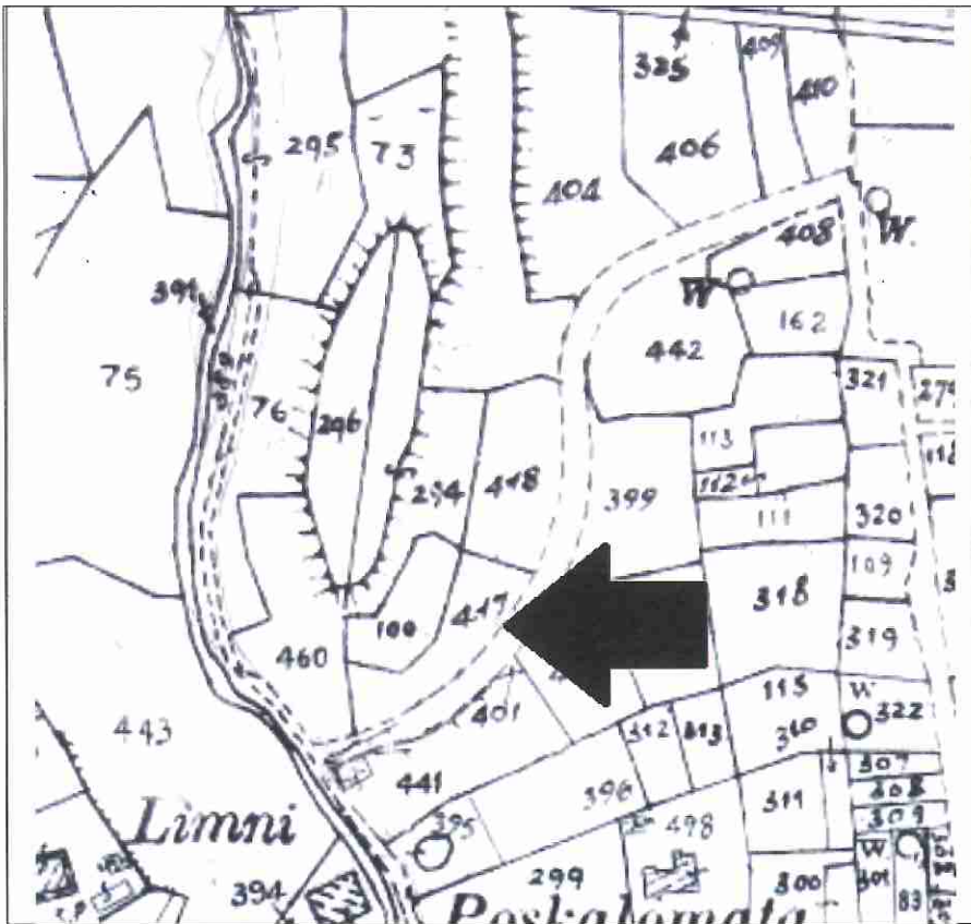
Χωρομετρικό Σχέδιο.
