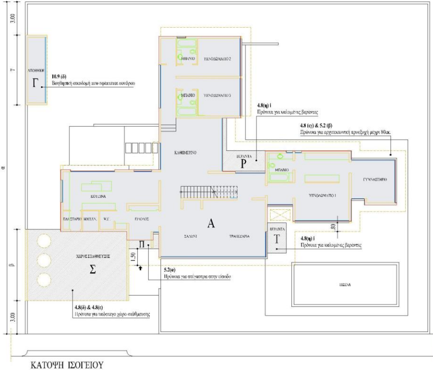
ΚΑΤΩΨΗ ΙΣΟΓΕΙΟΥ
